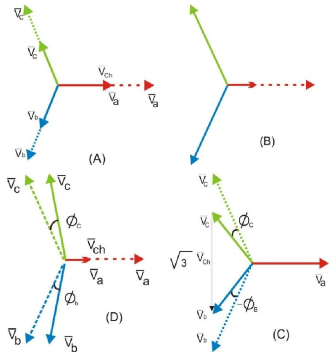
Fig. 3.Types of Sag
